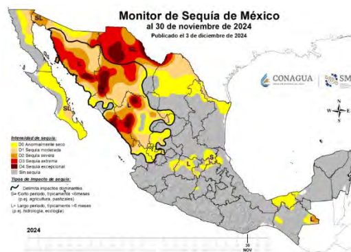
Monitor de sequía de la CONAGUA
