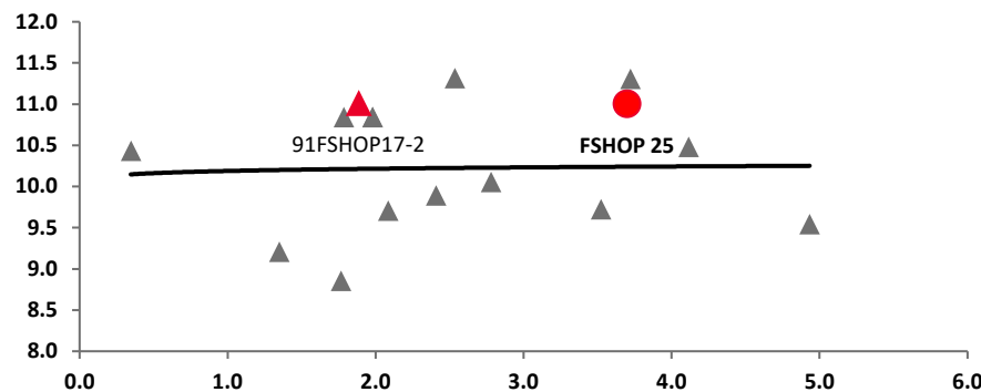
FSHOP 25 – Fija Duración vs. YTM (%)
