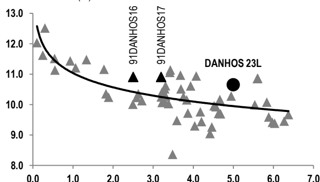
DANHOS 23L – Fija Duración vs. YTM (%)
