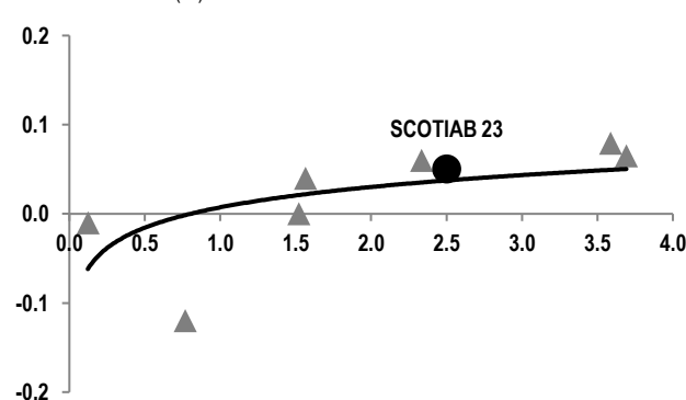
SCOTIAB 23 – TIIE-28 AxV vs. Sobretasa (%)
