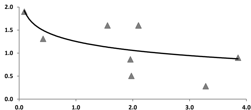
CEMEX 23L – TIIE-28 AxV vs. Sobretasa (%)
